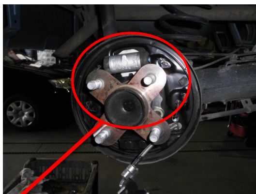
④リヤブレーキ点検・整備
