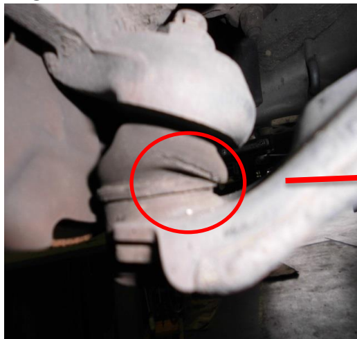
⑤ロアボールジョイントブーツ亀裂有
