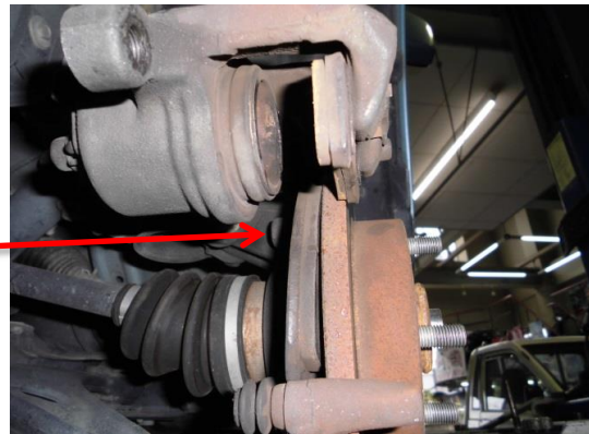
②ブレーキパッドの点検・清掃・グリスアップ
